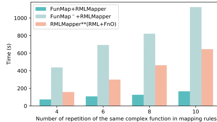
(d) RMLMapper - 75% of duplicates
